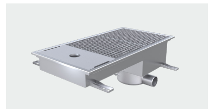
STÄDRUMSBRUNN FURO 325: Rostfri kvalitet EN 1.4301, sido- eller bottenutlopp, storlek 600 x 400 mm.
