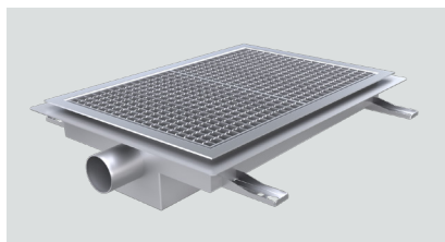
LÅG ROT-GOLVBRUNN FURO 123: Syrafast kvalitet EN 1.4404, sido- eller bottenutlopp, storlek 600 x 400 mm.
