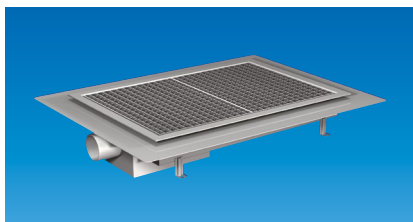
LAV REHAB-GULVSLUK FURO 123: Syrefast kvalitet EN 1.4404, side- eller bunnutløp, størrelse 600 x 400 mm.
