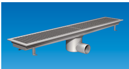
SMAL GULVRENNE FURO 115: Syrefast kvalitet EN 1.4404, side- eller bunn- utløp. Bredde 150 mm og lengde 800 mm, 900 mm, 1000 mm, 1100 mm, 1200 mm, 1300 mm, 1400 mm, 1500 mm og 2000 mm.
