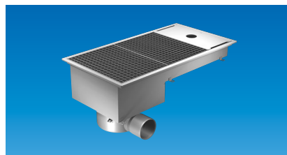
VASKEROMSBRØNN FURO 325: Rustfri kvalitet EN 1.4301, side- eller bunnutløp, størrelse 600 x 400 mm.
