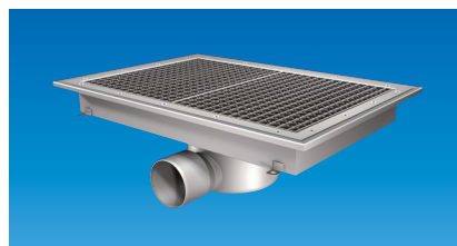
STORT GULVSLUK FURO 113: Syrefast kvalitet EN 1.4404, side- eller bunn- utløp, størrelse 300 x 300, 400 x 300 mm, 500 x 300 mm, 400 x 400 mm, 600 x 400 mm, 800 x 500 mm, 900 x 600 mm.
