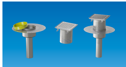
TERASSEBRØNN FURO 191, 192: Syrefast kvalitet EN 1.4404, bunnutløp.
