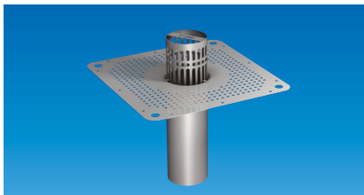
TAKSLUK FURO 180, 182: Rustfri kvalitet EN 1.4301, bunnutløp.
