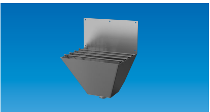
UTSLAGSVASK FR 318: Rustfri kvalitet EN 1.4301.
