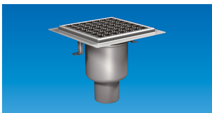
GULVSLUK FURO 104: Syrefast kvalitet EN 1.4404, side- eller bunnutløp.
